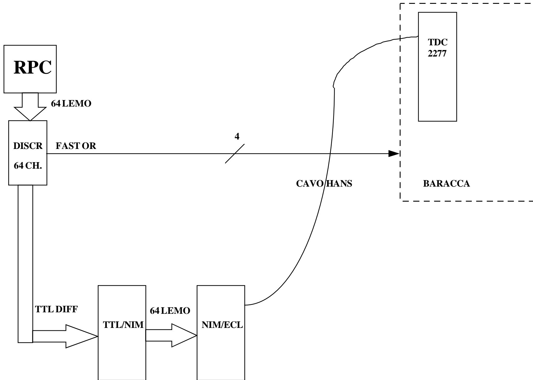
Nuova disposizione elettronica per test beam (I opzione)
